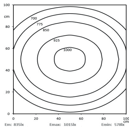
HELULIGHT® CLASSIC 1400 mm (11024037)
