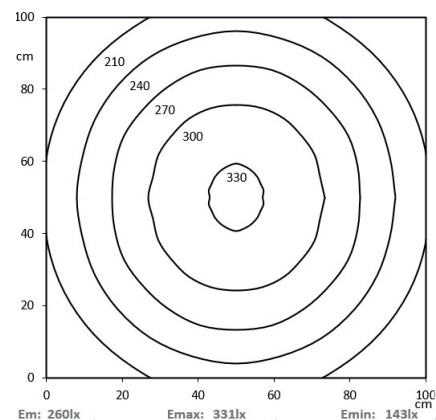
HELULIGHT® CLASSIC 420 mm (11024033, 11024040)
